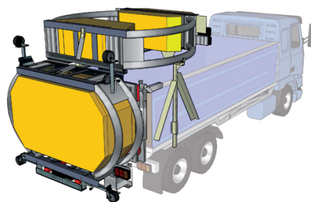
TMA-skydd Skorpionen, typ C
