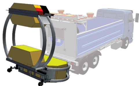
TMA-Skydd Skorpion, Typ B
